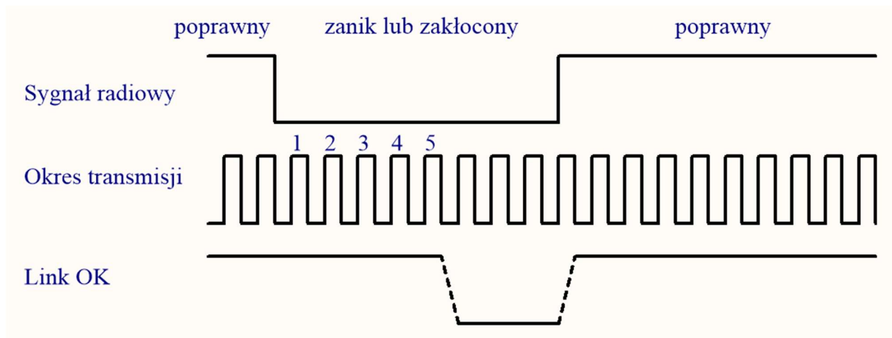
Rys. 4.2.1 Diagram działania wyjścia Link OK dla wartości Error cycle = 5
